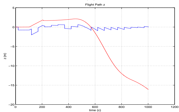
Рис. 2: Ошибки позиции ((a) для координаты x (b) для координаты y (c) для координаты z). Ошибки инерциального дрейфа отмечены красной линией, и ошибки, исправленные видео-навигацией, отмечены синей линией.
